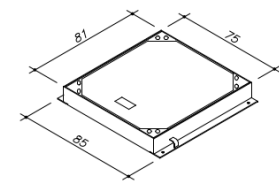
Abb.1 Beispiel Mönninghof Fertigbauteile KS 70/70
